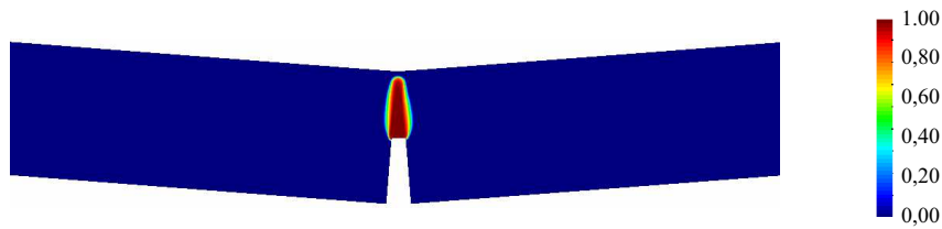
Figura A.9: Flexión de viga entallada con fuerzas en tres puntos. Mapa de la variable de daño d para un estado avanzado de degradación.
