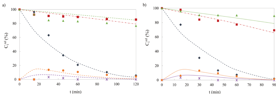
Figura 4.4. Resultados experimentales y del modelo para las concentraciones relativas de PCT, HP, Oxa, HQ y BQ. (a) Baja Rad, T = 50^\circ\text{C} , \text{HP} = 756 \text{ mg L}^{-1} ; (b) Alta Rad, T = 50^\circ\text{C} , \text{HP} = 189 \text{ mg L}^{-1} . Claves: líneas continuas: resultados del modelo y ( \diamond ) PCT, ( \blacksquare ) HP, ( \blacktriangle ) Oxa, ( \bullet ) HQ, and ( * ) BQ, resultados experimentales.
