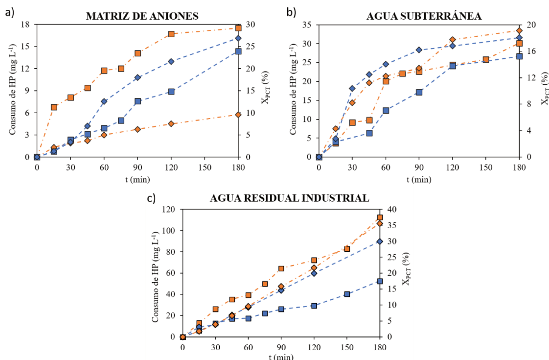
Figura 4.5. Evoluciones temporales del consumo de HP (en mg L -1 , símbolos = ■) y de la conversión de PCT (en %, símbolos = ◆) para ensayos realizados en diferentes matrices acuosas, RAD = ON, y HP = 378 mg L -1 . Los ensayos con dosificación de HP están en azul y con línea de guion-largo, y los ensayos sin dosificación de HP están en naranja y con línea guion-punto.
