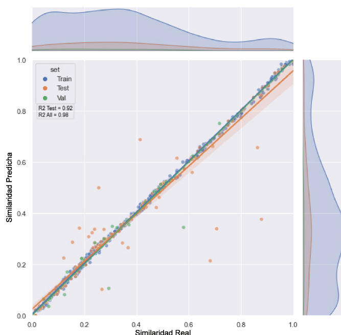
Figura 4.5: Comparación entre la similitud de Tanimoto real y predicha. R^2 indica el coeficiente de correlación de Pearson al cuadrado para el conjunto de prueba y para todo el conjunto de datos, respectivamente. Los valores de entrenamiento se muestran en azul, los valores de prueba en naranja y los valores de validación en verde.
