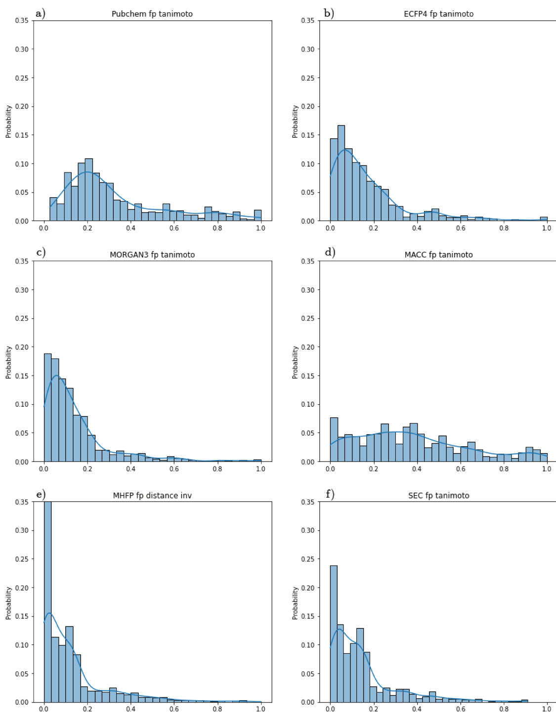
Figura 3.3: Histograma de la distribución de los valores de similaridad calculado con el índice de Tanimoto para las diferentes fingerprints consideradas sobre el camino metabólico de la Glucólisis: a) Pubchem, b) ECFP de radio 4, c) MORGAN (radio 3), d) MACCS, e) MHFP, f) SEC
