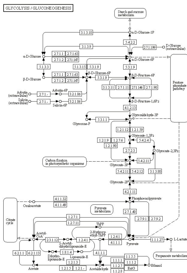
Figura 1.1: Representación del camino metabólico de la glucólisis/gluconeogénesis obtenido de la base de datos KEGG. Los compuestos químicos (metabolitos) aparecen como nodos circulares, mientras que las reacciones enzimáticas —identificadas por sus números EC— conectan sustratos con productos. Esta estructura ilustra cómo las vías metabólicas pueden modelarse naturalmente como grafos, donde la topología de la red refleja las relaciones bioquímicas entre compuestos. Las conexiones con otros caminos metabólicos (ciclo de Krebs, vía de las pentosas fosfato, metabolismo del piruvato) evidencian la naturaleza interconectada del metabolismo celular.
