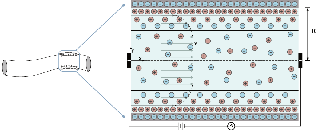
Figura 4.1: Representación esquemática del desplazamiento de la doble capa eléctrica bajo la acción de un campo eléctrico externo en un capilar. (Imagen inspirada en Gao et al. [2024])
