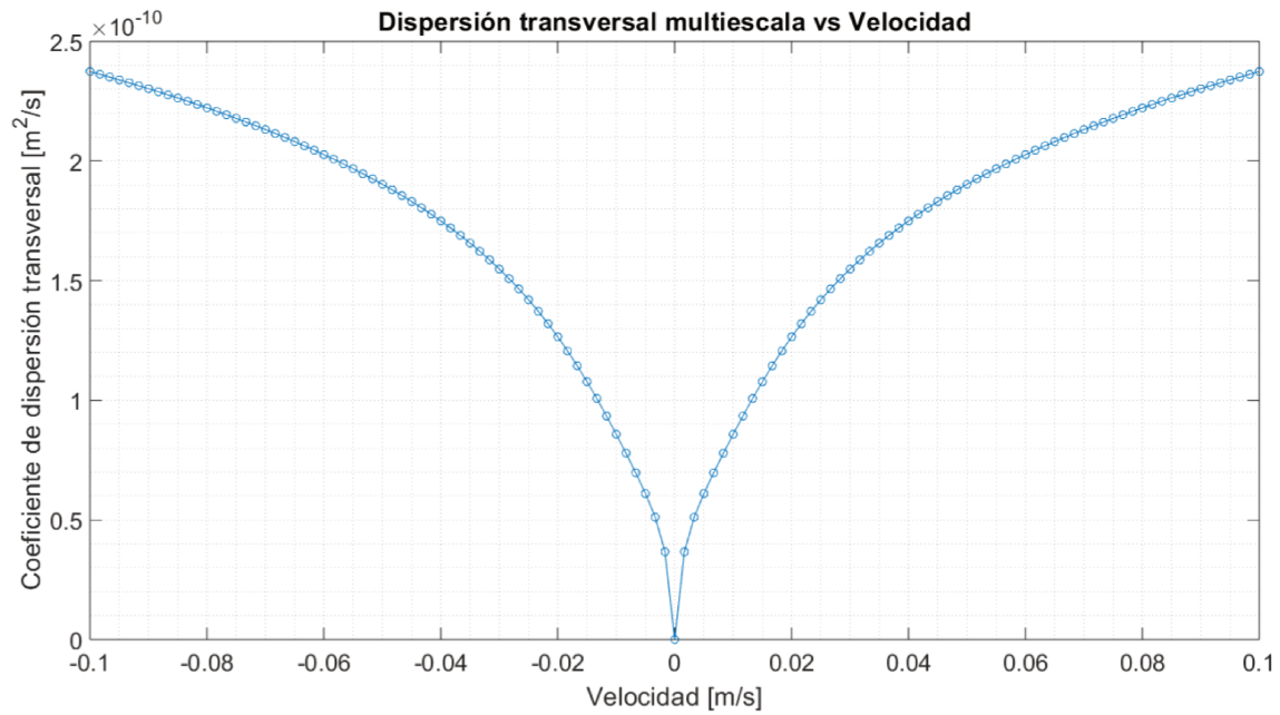
(b) Coeficiente de dispersión transversal.
