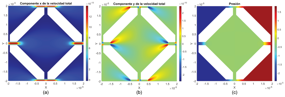
Figura 3.9: Solución del problema de flujo en la microescala para la geometría propuesta del papel Whatman #1: (a) Componente de la velocidad en la dirección x ; (b) Componente de la velocidad en la dirección y ; y (c) Campo de presión.
