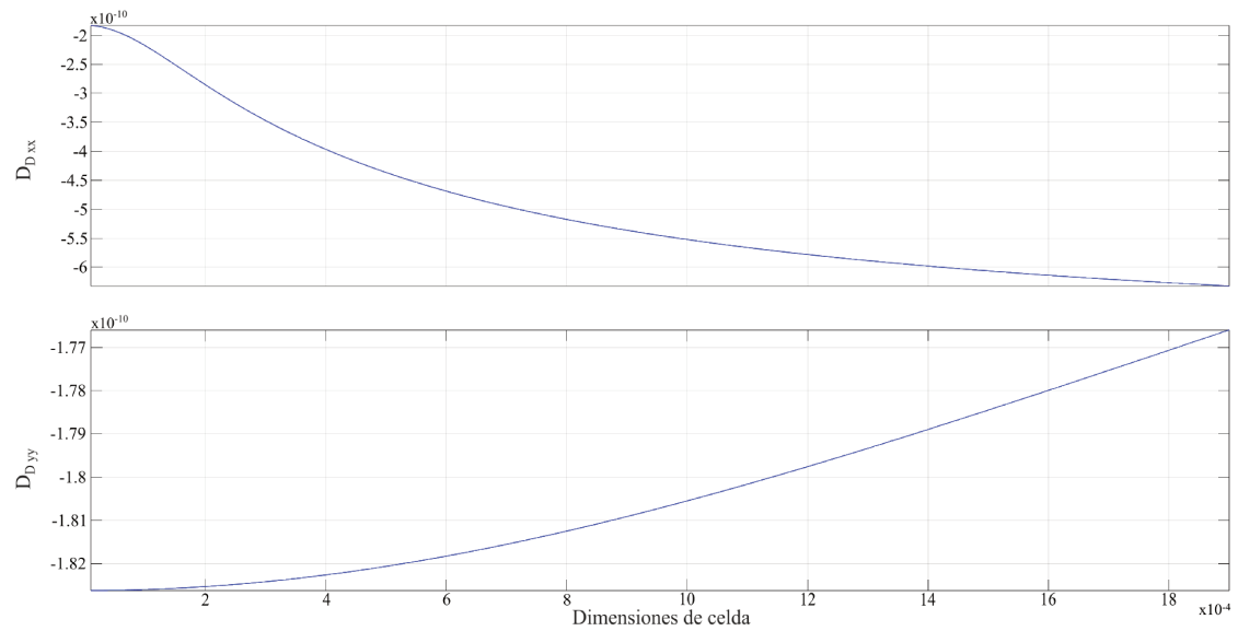
Figura 5.9: Análisis de sensibilidad de D_{Dxx} y D_{Dyy} del tensor de difusividad efectivo con las dimensiones de la microcelda.
