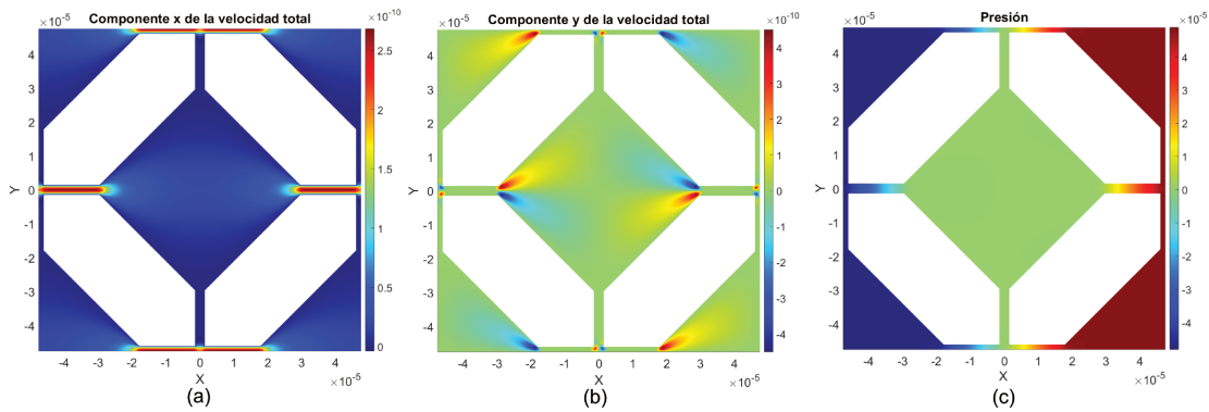
Figura 3.8: Solución del problema de flujo en la microescala para la geometría propuesta del papel Munktell 00A: (a) Componente de la velocidad en la dirección x ; (b) Componente de la velocidad en la dirección y ; y (c) Campo de presión.
