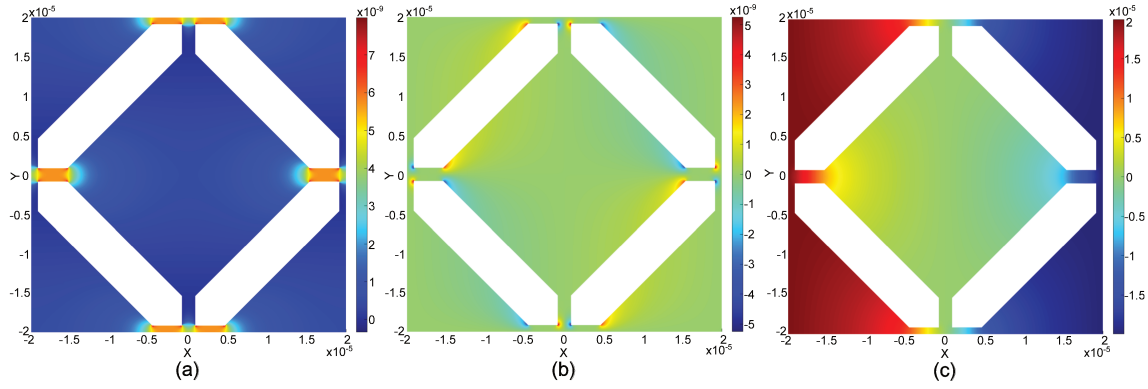
Figura 4.4: Solución del problema de flujo electroosmótico en la microescala para geometría Whatman #1 mediante el modelo multiescala propuesto: (a) Campo de velocidades en dirección tangencial al flujo; (b) Campo de velocidades en dirección perpendicular al flujo; (c) Campo potencial eléctrico.
