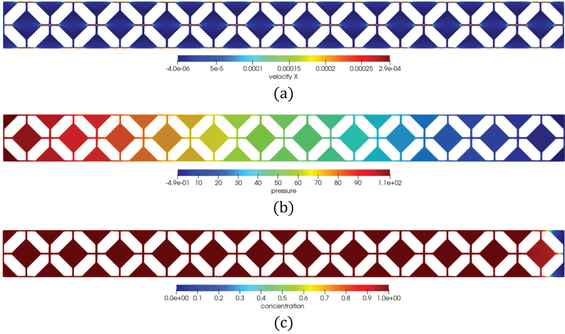
Figura 5.11: Soluciones obtenidas por simulación numérica directa (DNS) del problema de Transporte Escalar para papel Munktell 00A: (a) Velocidad tangencial al flujo; (b) Campo de presiones; (c) Campo de Concentración.
