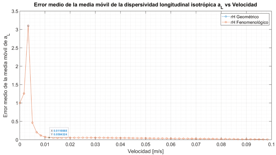
(a) Error medio de la media móvil de la dispersividad longitudinal.
