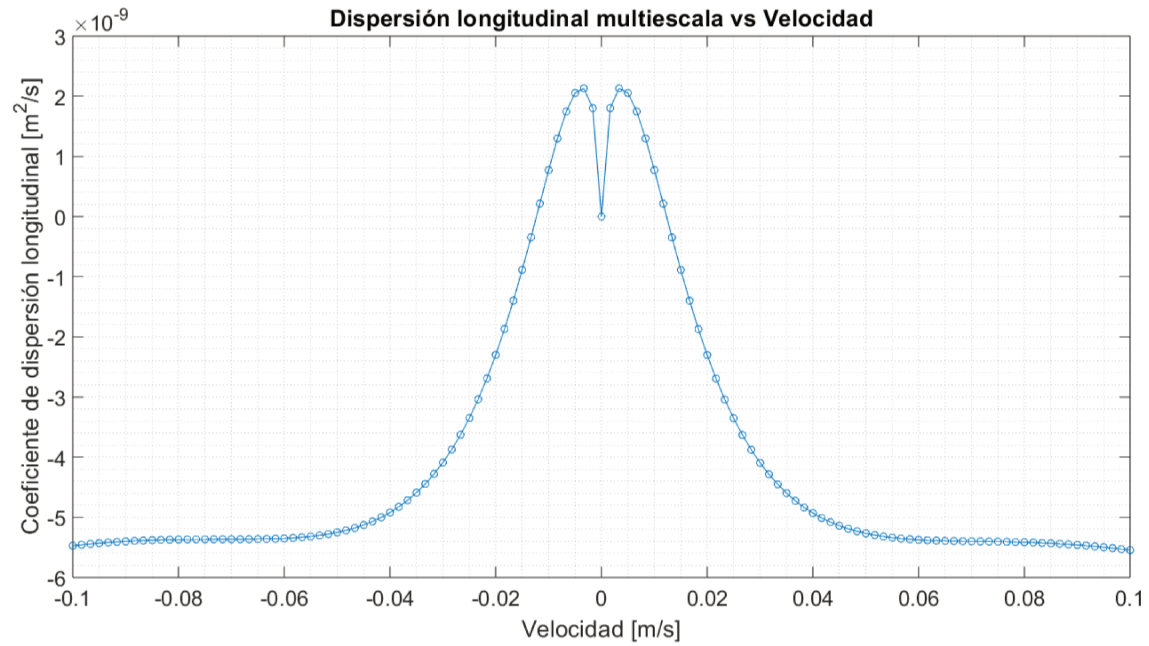
(a) Coeficiente de dispersión longitudinal.
